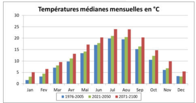
Température médianes mensuelles de la période de référence et variations de températures pour le futur proche et le futur lointain
